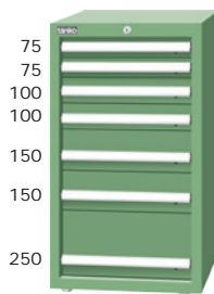
EA-10073 H1000xW566xD607 72pcs/20ft ; 152pcs/40ft EB-10073 H1000xW718xD607 54pcs/20ft ; 114pcs/40ft ED-10073 H1000xW718xD759 42pcs/20ft ; 90pcs/40ft
