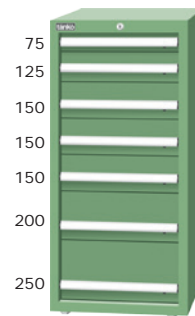
EA-12073 H1200xW566xD607 36pcs/20ft ; 76pcs/40ft EB-12073 H1200xW718xD607 27pcs/20ft ; 57pcs/40ft ED-12073 H1200xW718xD759 21pcs/20ft ; 45pcs/40ft
