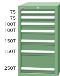
EA-10073T H1000xW566xD607 72pcs/20ft ; 152pcs/40ft EB-10073T H1000xW718xD607 54pcs/20ft ; 114pcs/40ft ED-10073T H1000xW718xD759 42pcs/20ft ; 90pcs/40ft
