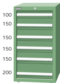
EA-10062 H1000xW566xD607 72pcs/20ft ; 152pcs/40ft EB-10062 H1000xW718xD607 54pcs/20ft ; 114pcs/40ft ED-10062 H1000xW718xD759 42pcs/20ft ; 90pcs/40ft
