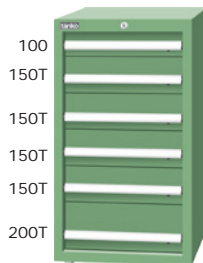
EA-10062T H1000xW566xD607 72pcs/20ft ; 152pcs/40ft EB-10062T H1000xW718xD607 54pcs/20ft ; 114pcs/40ft ED-10062T H1000xW718xD759 42pcs/20ft ; 90pcs/40ft
